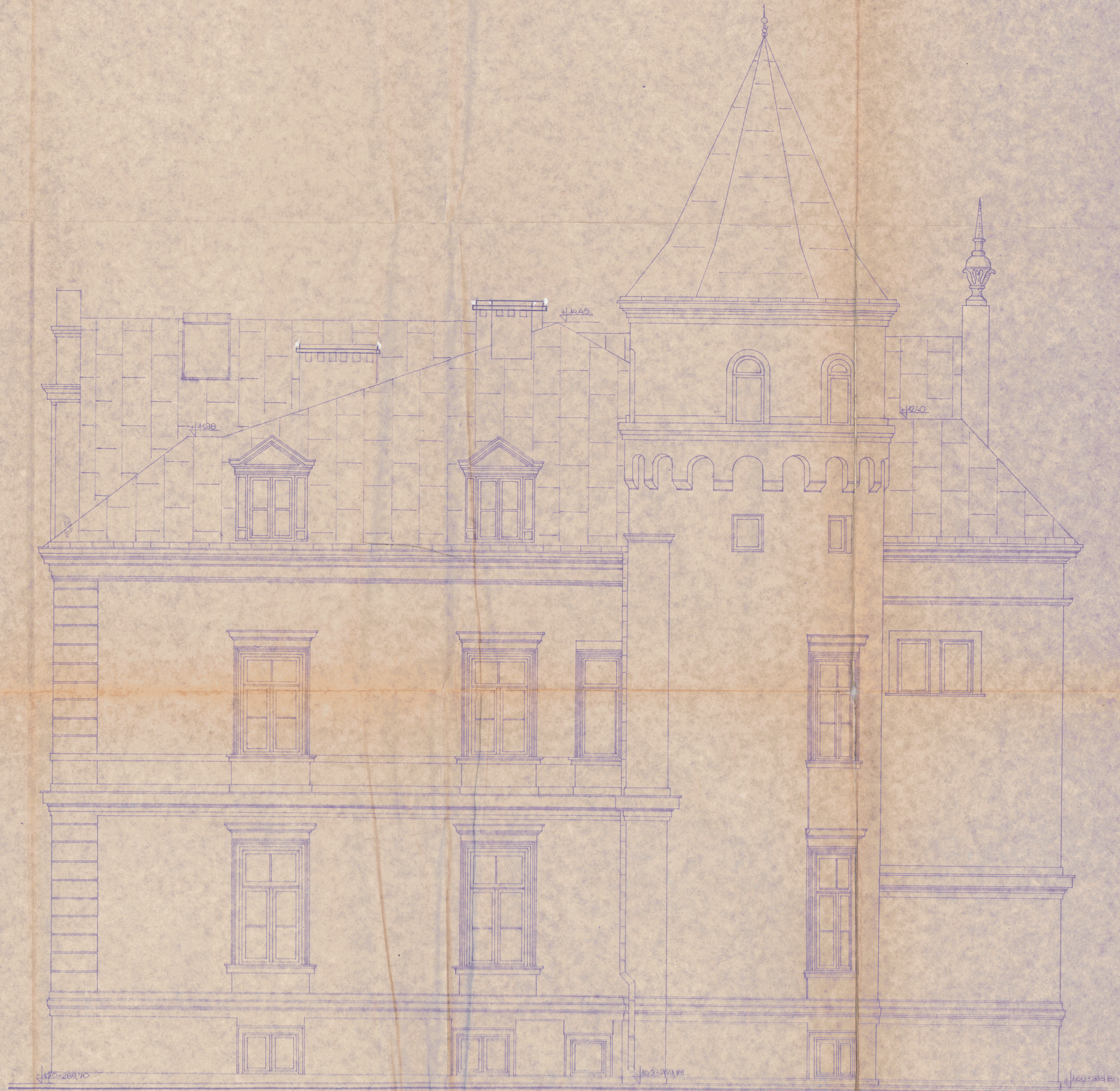
ELEWACJA WSCHODNIA .150.
